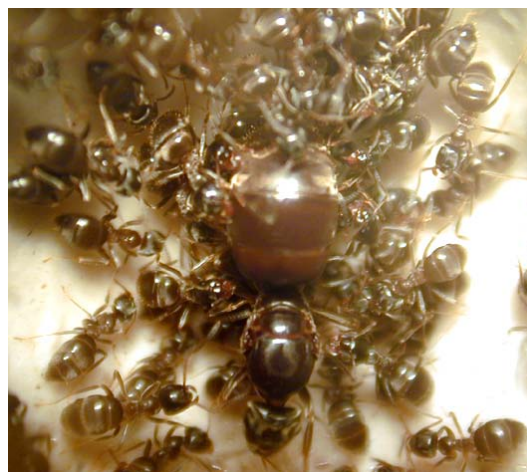
Hormiga común (Lasius niger) y reina
